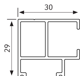
Führungsschiene ZIP 30/29 einfach
