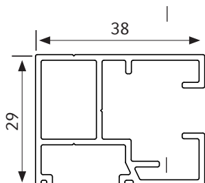
Führungsschiene ZIP 38/29 einfach
