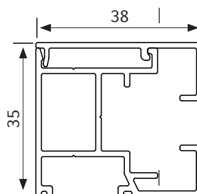
Führungsschiene ZIP 38/35, 2-teilig Linksroller einfach
