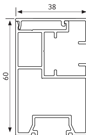
Führungsschiene ZIP 38/60, 2-teilig tiefe Ausführung einfach
