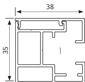
Führungsschiene ZIP 38/35, 2-teilig Rechtsroller einfach
