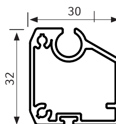
Endschiene 32 mm, max. Breite 3000 mm
