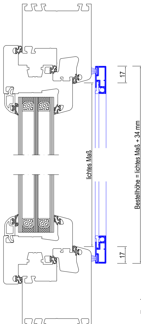
Vertikalschnitt
