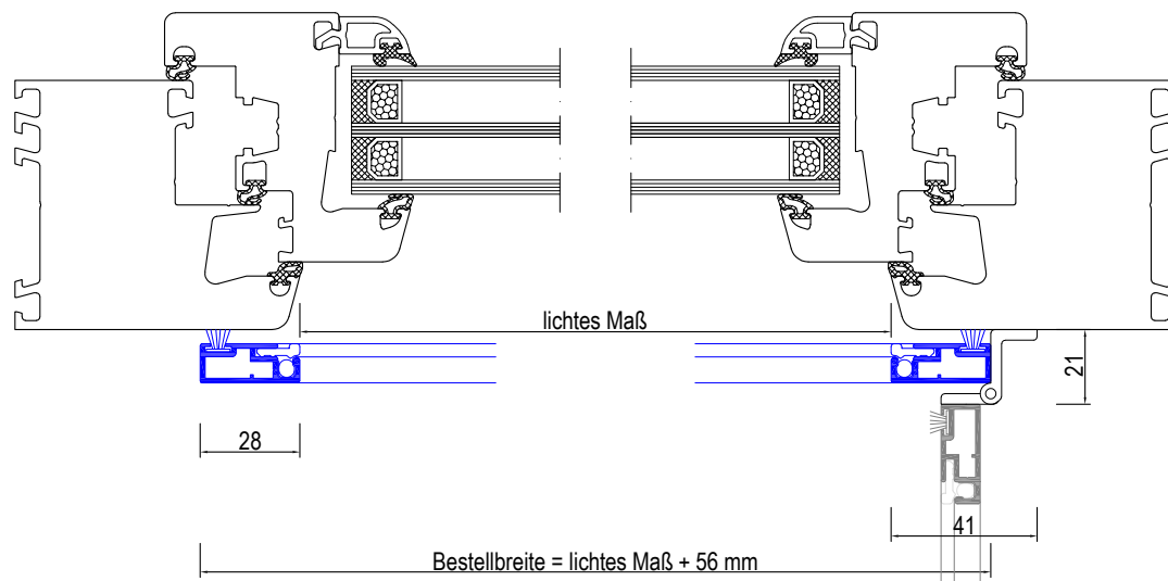
Vertikalschnitt
