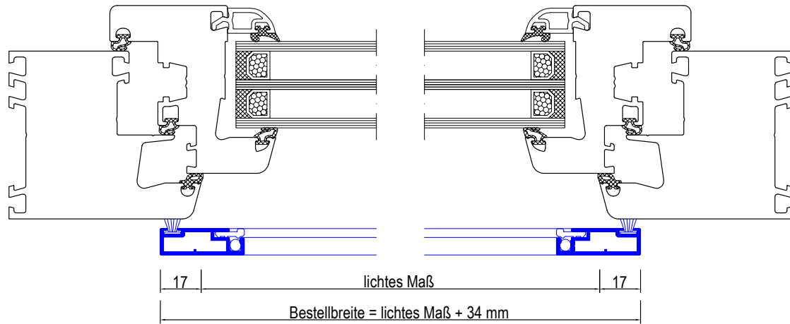
Vertikalschnitt
