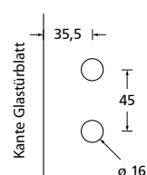
Bohrmaße 3-teiliges Band
