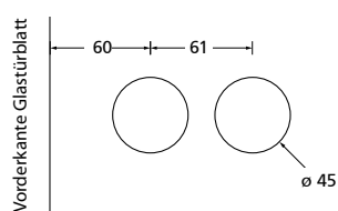
Bohrmaße Glastürschloss
