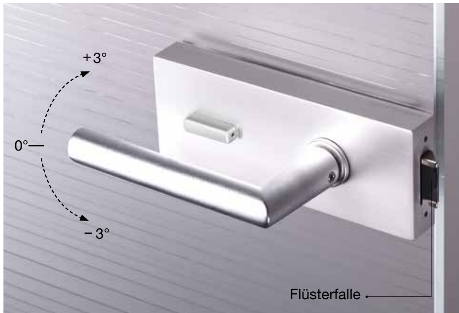
Schlosskasten Edge mit WC-Verriegelung offen und Drücker vorne, F1 Aluminium
